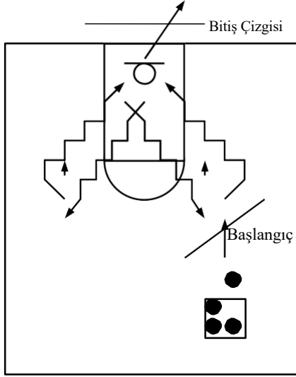
Şekil 4. Turnike testi
