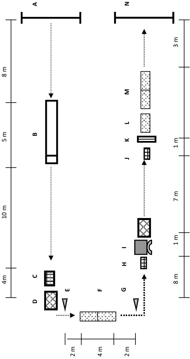
Şekil 2. Koordinasyon Testi
