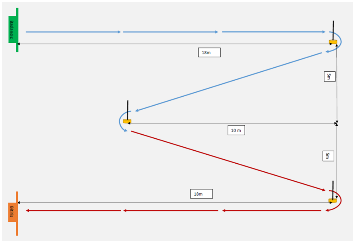
Şekil 5. Özel Gereksinimi Olan (Engelli) Aday Test Parkuru
