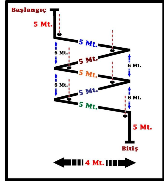
Şekil 1. Zikkaz Testi (Serpentine Çeviklik Testi).
