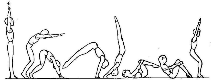
Şekil 1: Öne takla yuvarlanışı yapılırken, dönüşü yavaşlatacağı için kesinlikle dizler göğüse çekilmez.
